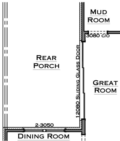
12' Sliding Door
