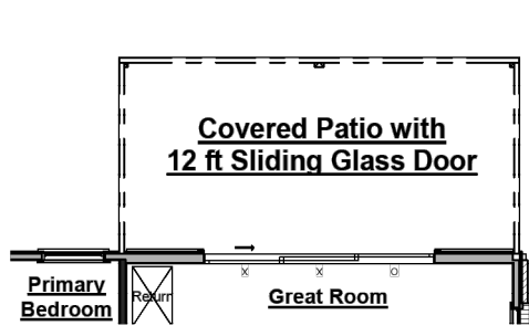
12ft Sliding Glass Door
