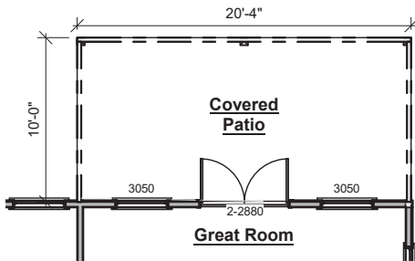
Double Door
